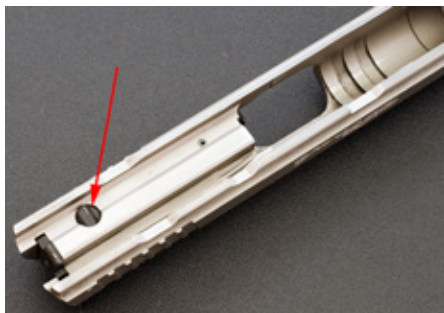
Tanfoglio Stock III har en passiv säkring i form av ett slagstiftslås.
