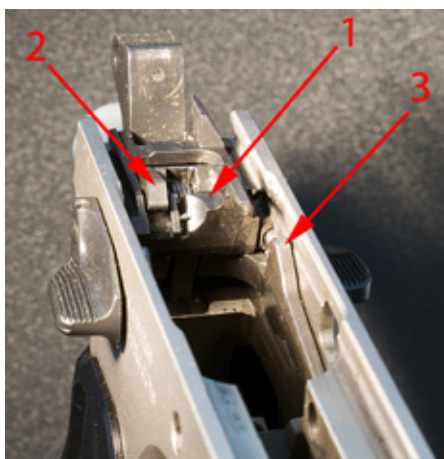
Urverket hos Tanfoglio Stock III
